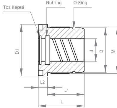
KESİT(SECT.) A-A
