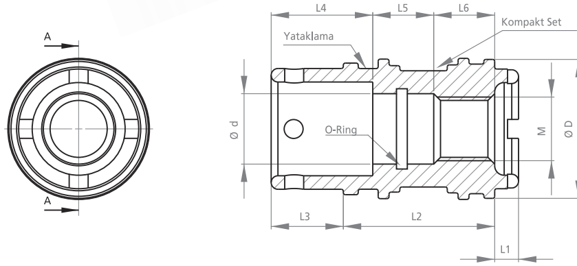
KESİT(SECT.) A-A
