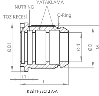
KESİTT(SECT.) A-A
