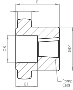
POMPA MİLİNE GÖRE İŞLENMİŞ KAPLINLER PROCESSED COUPLINGS PUMP SHAFT
