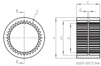
KESİT (SECT) B-B
